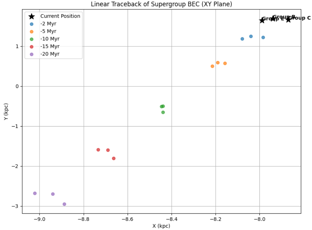
FIGURE 13 – Traceback linéaire des amas d'étoiles du super-groupe BEC selon le plan galactique. L'axe des abscisses représente la distance au centre galactique, et l'axe des ordonnées représente la tangente à la trajectoire de rotation moyenne de la galaxie au niveau du Cygne.
