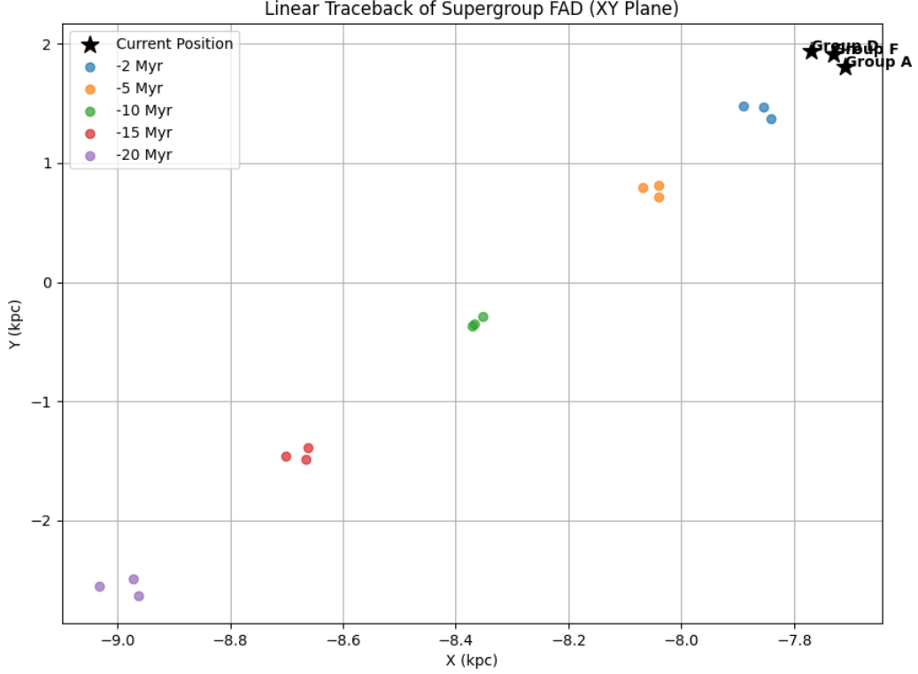
FIGURE 14 – Traceback linéaire des amas d'étoiles du super-groupe FAD selon le plan galactique. L'axe des abscisses représente la distance au centre galactique, et l'axe des ordonnées représente la tangente à la trajectoire de rotation moyenne de la galaxie au niveau du Cygne.
